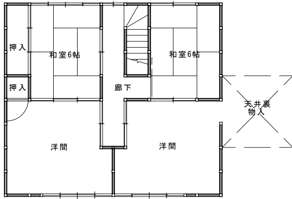
2階平面図
