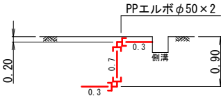
A 詳細図
