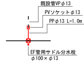
S1 給水工詳細図 土工2-2 0.65-13 L=1.0m L=1.0m×N=1
