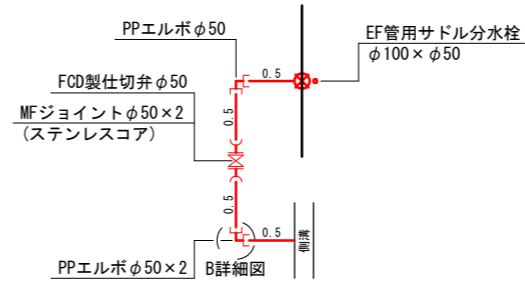
ドレーン工1詳細図 土工1-2 0.65-50 L=2.0m L=2.8m×N=1
