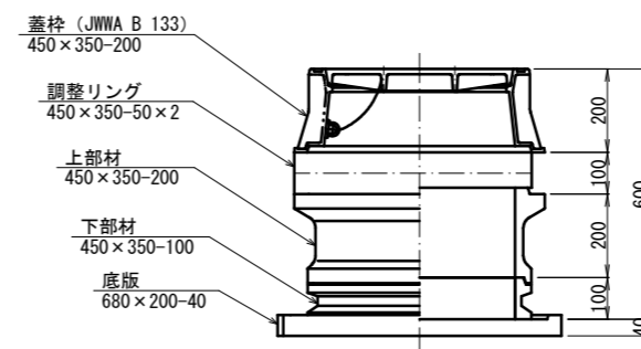
空気弁ボックス標準図
