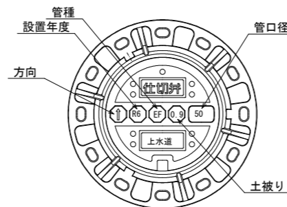
仕切弁筐 (鉄蓋) 参考図
