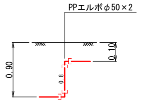
B詳細図
