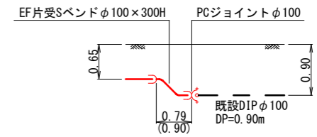
A詳細図
