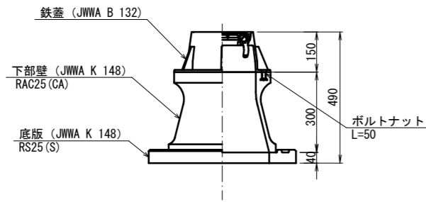
仕切弁筐標準図
