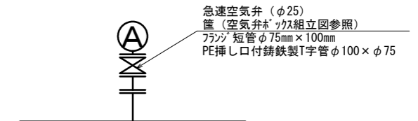
(空気弁工法図)
