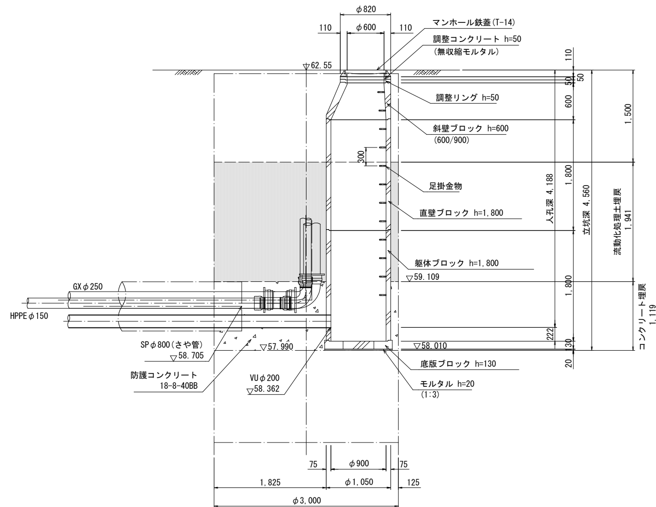
①-① 断面图
