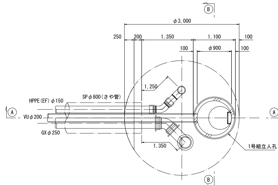
平面图
