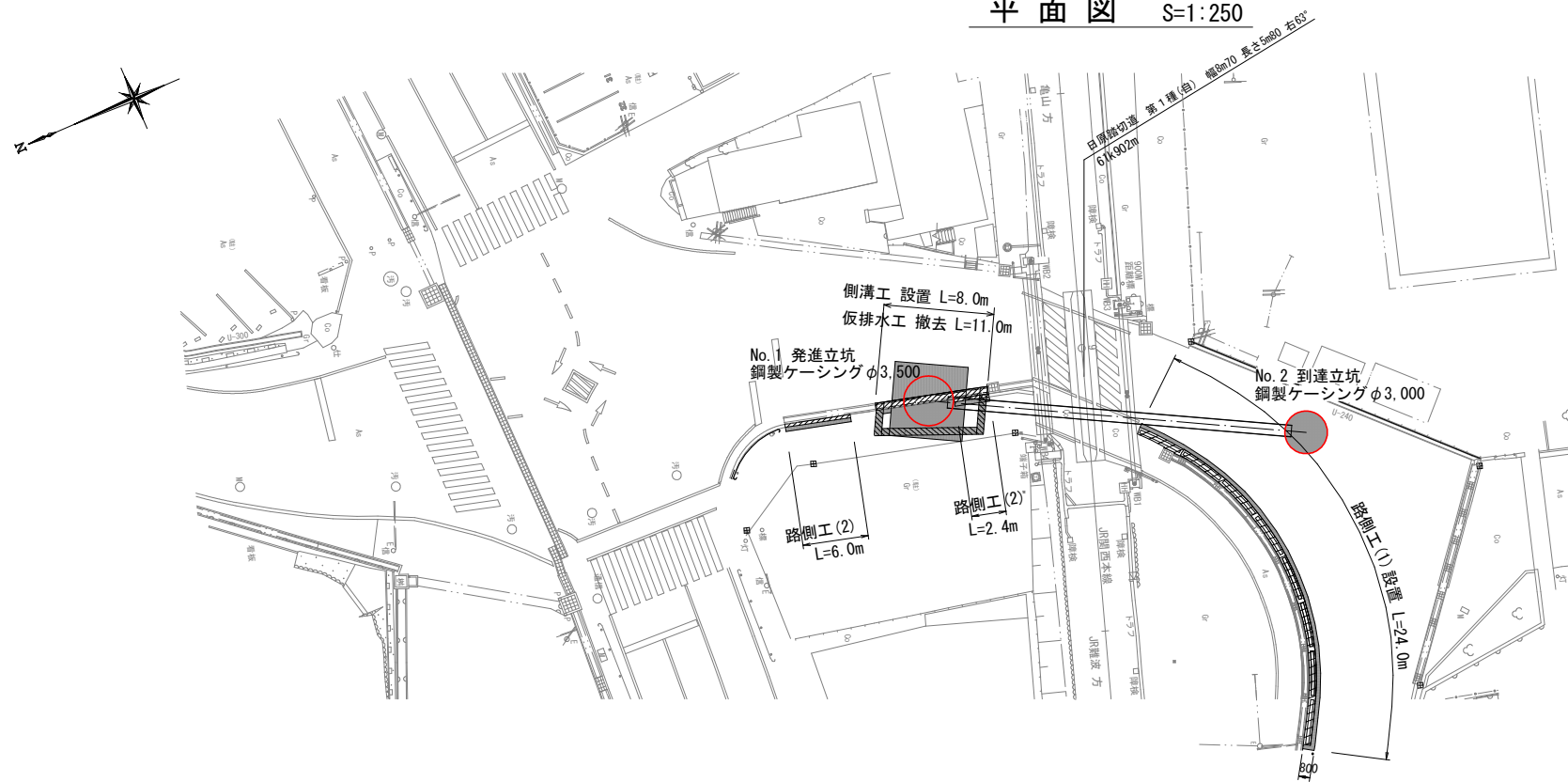
平面図 S=1:250
