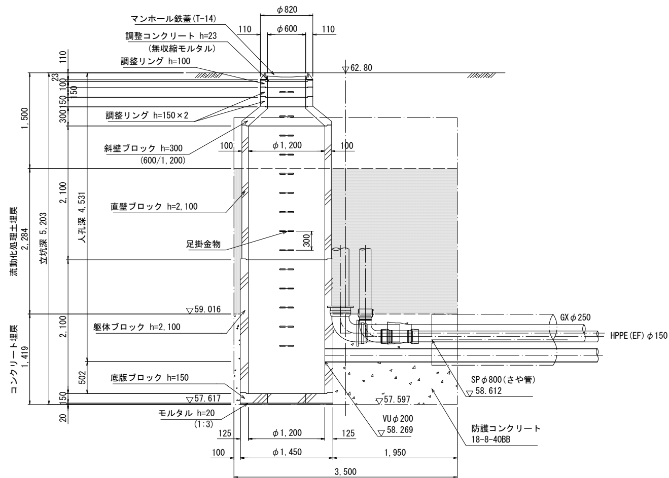
①-① 断面图
