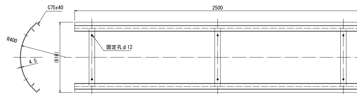
ガイドルール S=1:10
