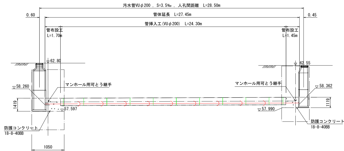
縦断図
