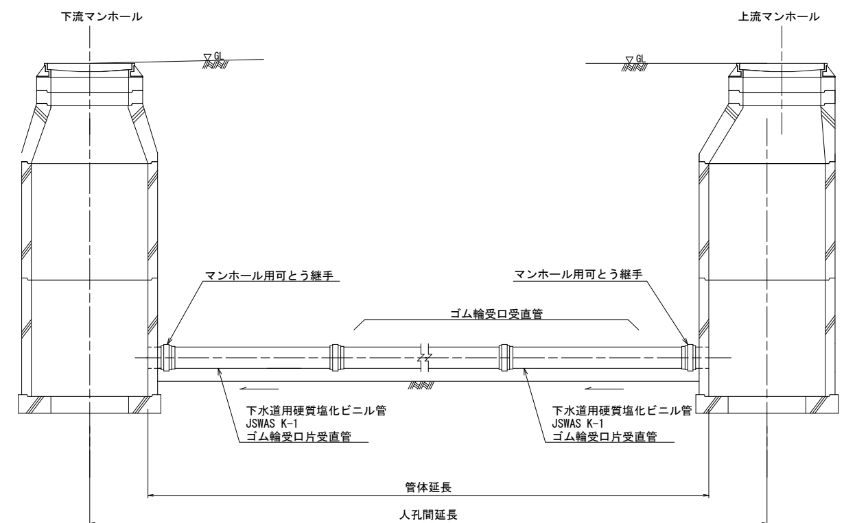
断面図
