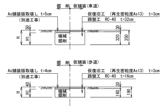
S=1:20
