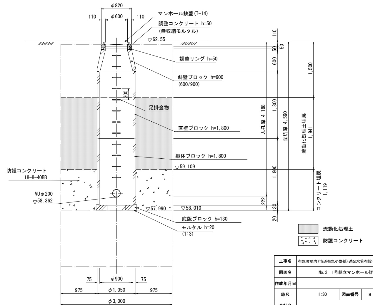
③-③ 断面图
