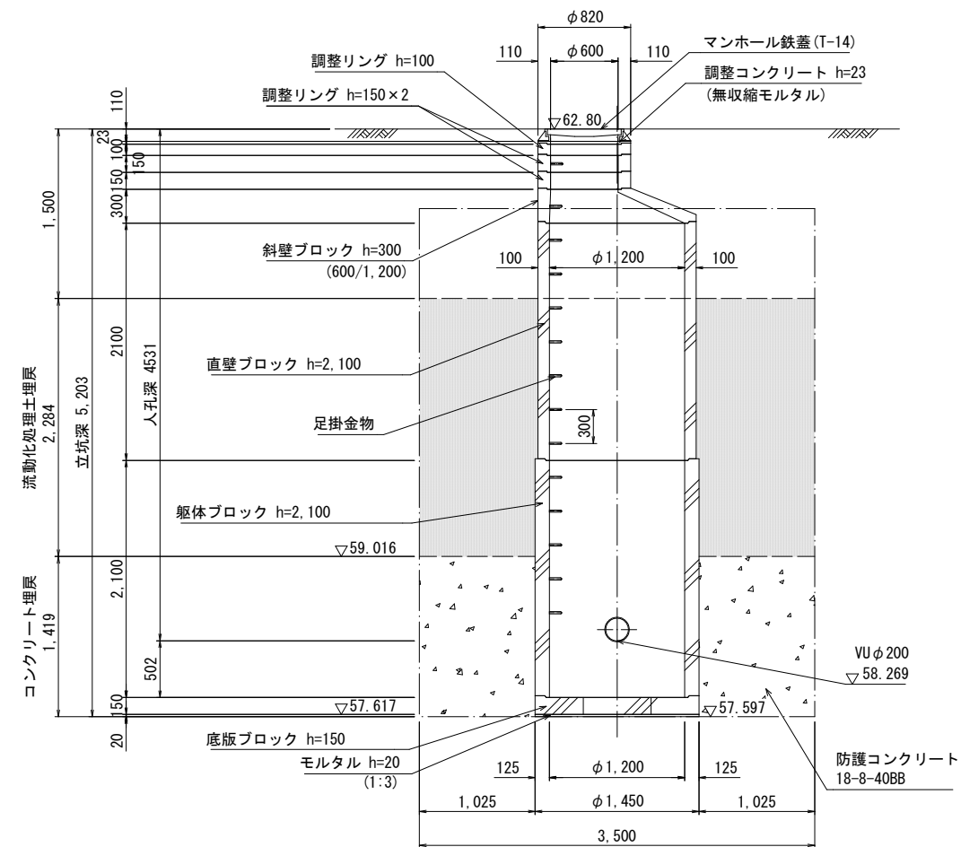
③-③ 断面图
