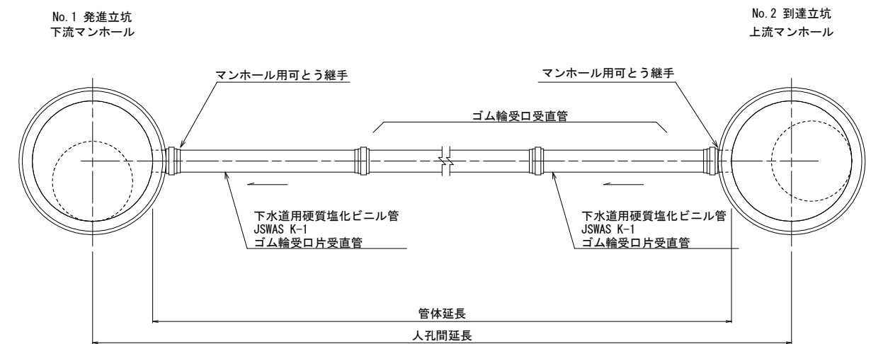
平面图
