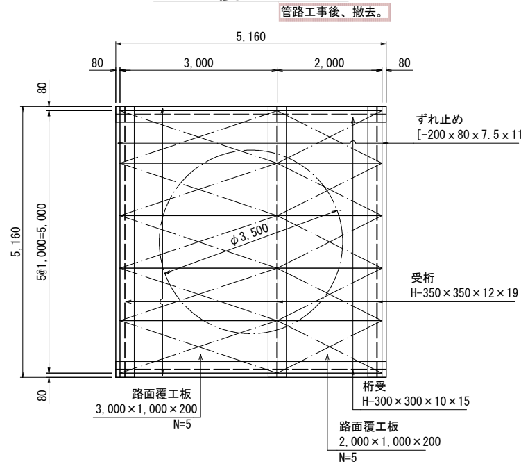
路面覆工平面図
