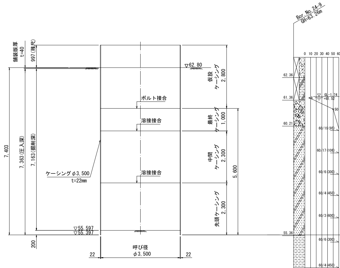
圧入掘削完了図 (別途工事)
