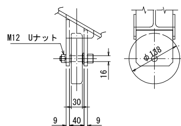
使用車輪
