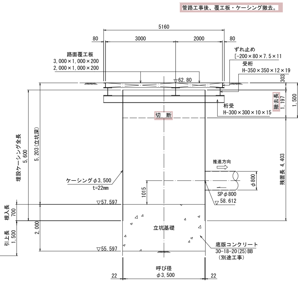
立坑基礎打設・引抜完了図
