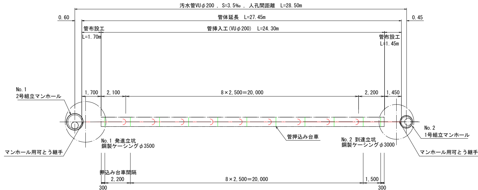
平面図
