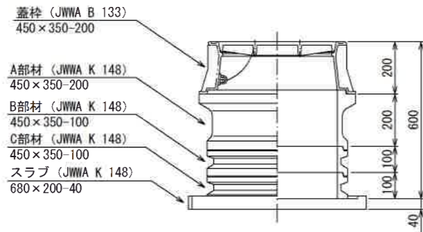
(消火栓工法図)
