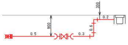
排泥断面図
