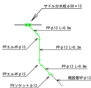
※13 仮設給水工詳細図 N=1 仮設1-11 0.3-13 L=1.4m
