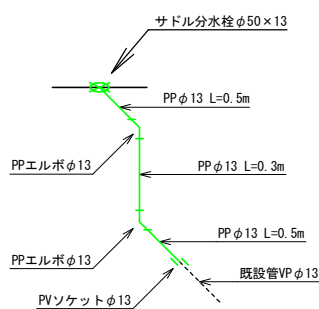
※12 仮設給水工詳細図 N=1 仮設1-11 0.3-13 L=1.0m
