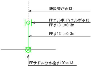
※1 仮設給水工詳細図 N=4 仮設1-11 0.3-13 L=0.3m
