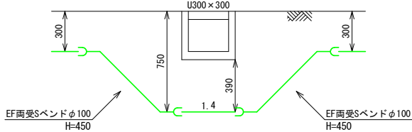
E - E' 断面図
