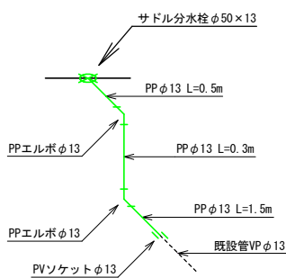
※8 仮設給水工詳細図 N=1 仮設1-11 0.3-13 L=2.0m
