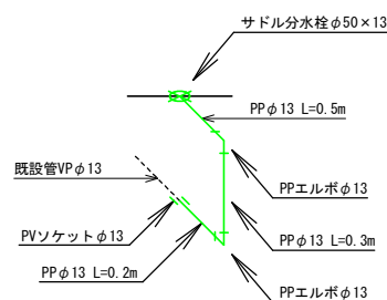
※7 仮設給水工詳細図 N=1 仮設1-11 0.3-13 L=0.5m
