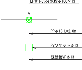
※3 仮設給水工詳細図 N=6 仮設1-11 0.3-13 L=2.0m
