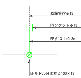
※5 仮設給水工詳細図 N=5+1 仮設1-11 0.3-13 L=0.3m
