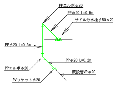
※10 仮設給水工詳細図 N=1 仮設1-10 0.3-20 L=0.5m
