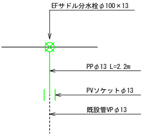
※6 仮設給水工詳細図 N=5 仮設1-11 0.3-13 L=2.2m
