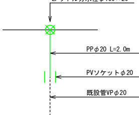
※4 仮設給水工詳細図 N=3 仮設1-10 0.3-20 L=2.0m
