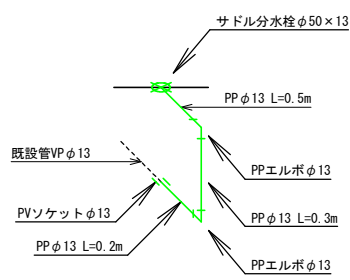
※14 仮設給水工詳細図 N=2 仮設1-11 0.3-13 L=0.5m
