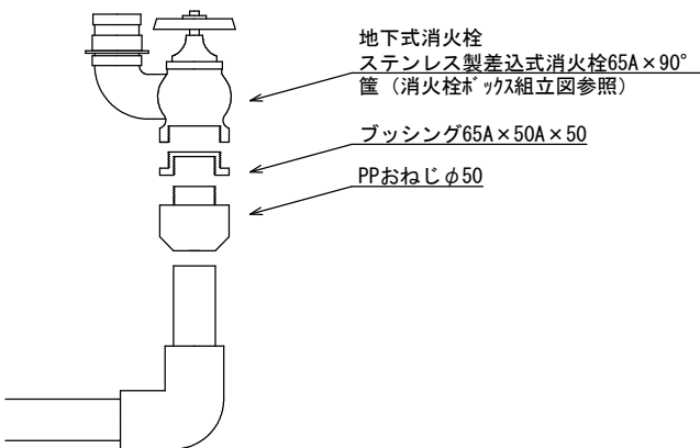
消火栓工法図 (PP)
