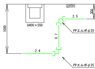
D - D' 断面図
