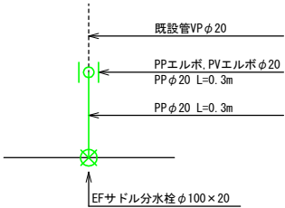
※2 仮設給水工詳細図 N=2 仮設1-10 0.3-20 L=0.3m
