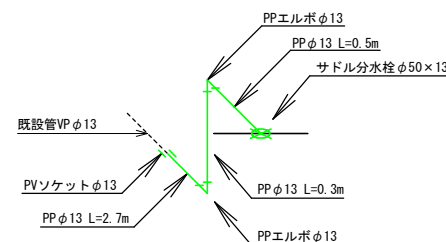
※15 仮設給水工詳細図 N=1 仮設1-11 0.3-13 L=3.2m
