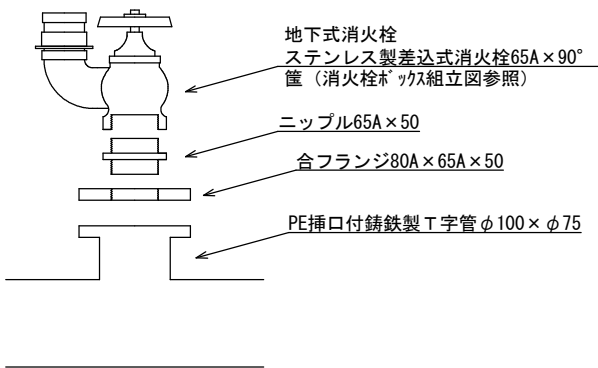
消火栓工法図 (HPPE)
