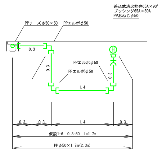
※消火栓詳細図
