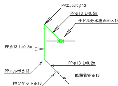
※11 仮設給水工詳細図 N=2 仮設1-11 0.3-13 L=0.5m
