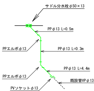
※9 仮設給水工詳細図 N=1 仮設1-11 0.3-13 L=4.9m
