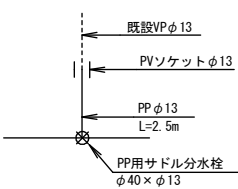
S5' 給水工詳細図 ±E1-4 0.3-13 L=2.5m L=2.5m×N=1
