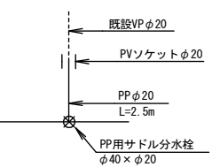
S7' 給水工詳細図 ±E2-3 0.3-20 L=5.0m L=2.5m×N=2
