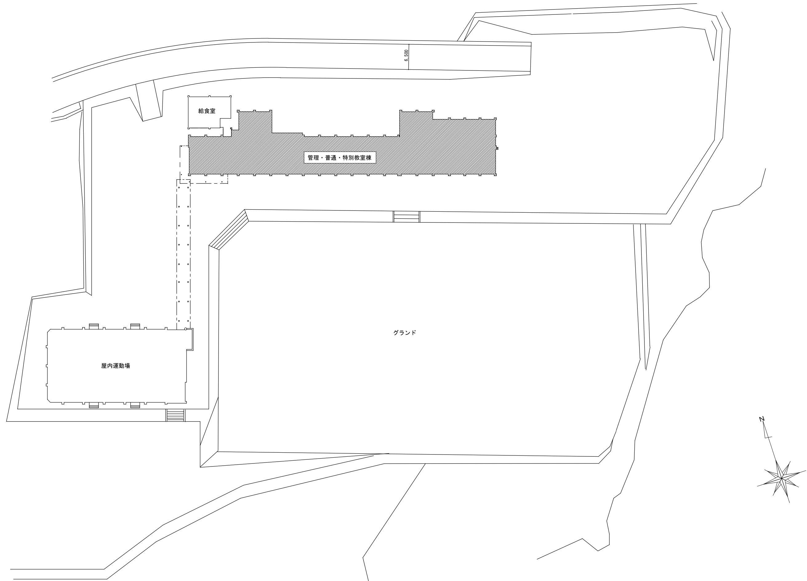
配置図 1/400
