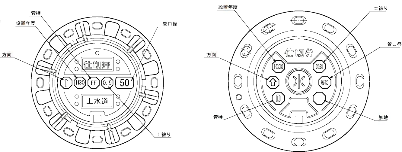
仕切弁箱 (鉄蓋) 参考図 S=Free
