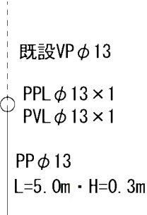
※16 給水工詳細図
