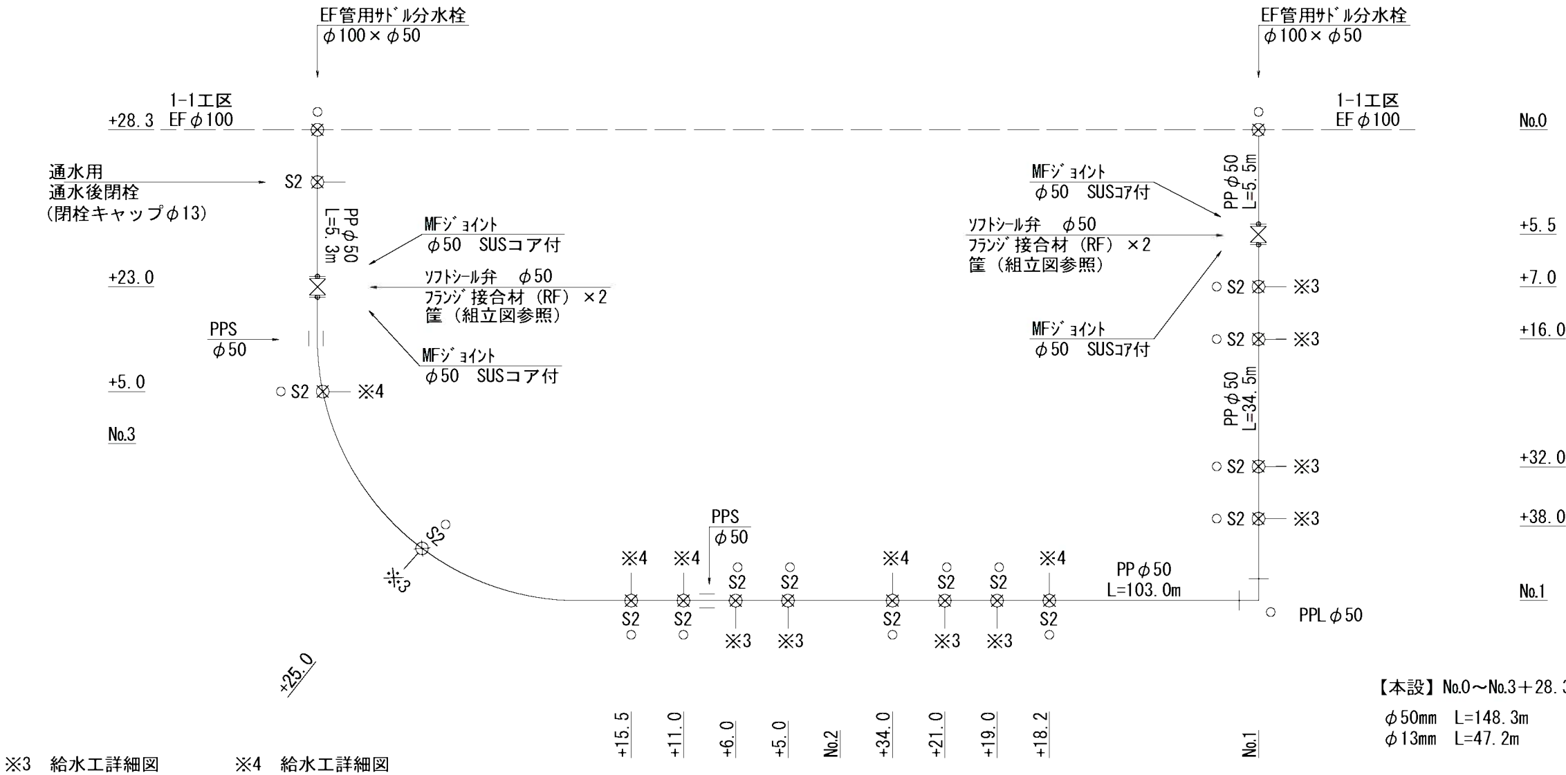
※3 給水工詳細図
