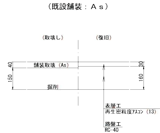
舗装構成 S=1:15
