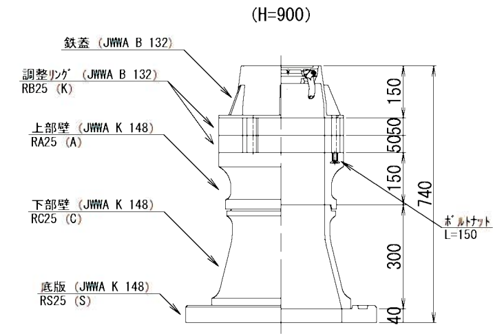
仕切弁設置部
