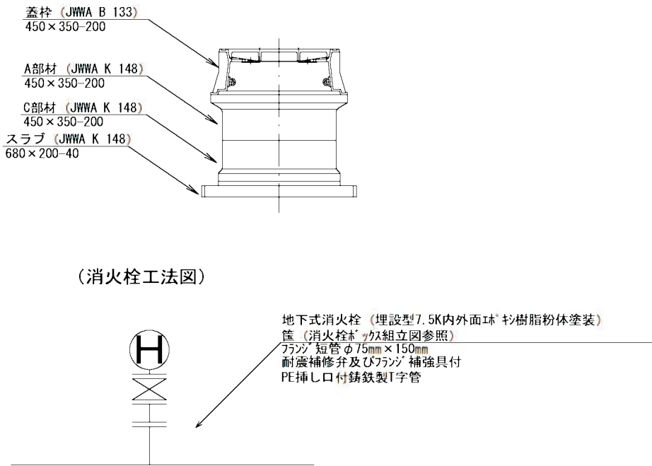
消火栓ボックス標準図 S=1:15
