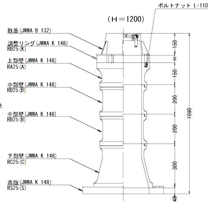
VP管用不断水ストップ設置部
