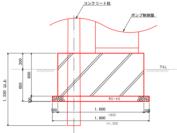
制御盤基礎図 S=1:20
