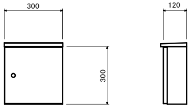
電話保安器箱 (ステンレス製)
