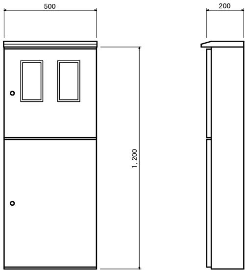
引込開閉器盤 (ステンレス製)
