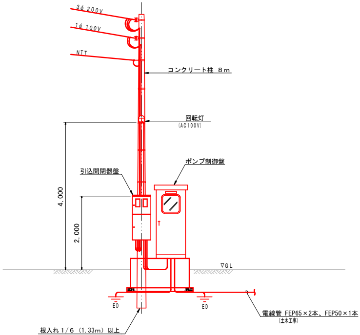
装柱図 S=1:50
