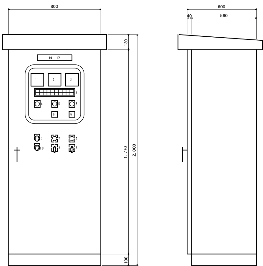
ポンプ制御盤 (ステンレス製)
