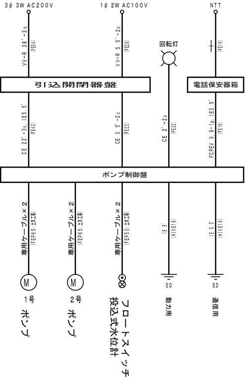
配線系統図
