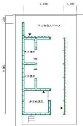
■ トイレ配置図
