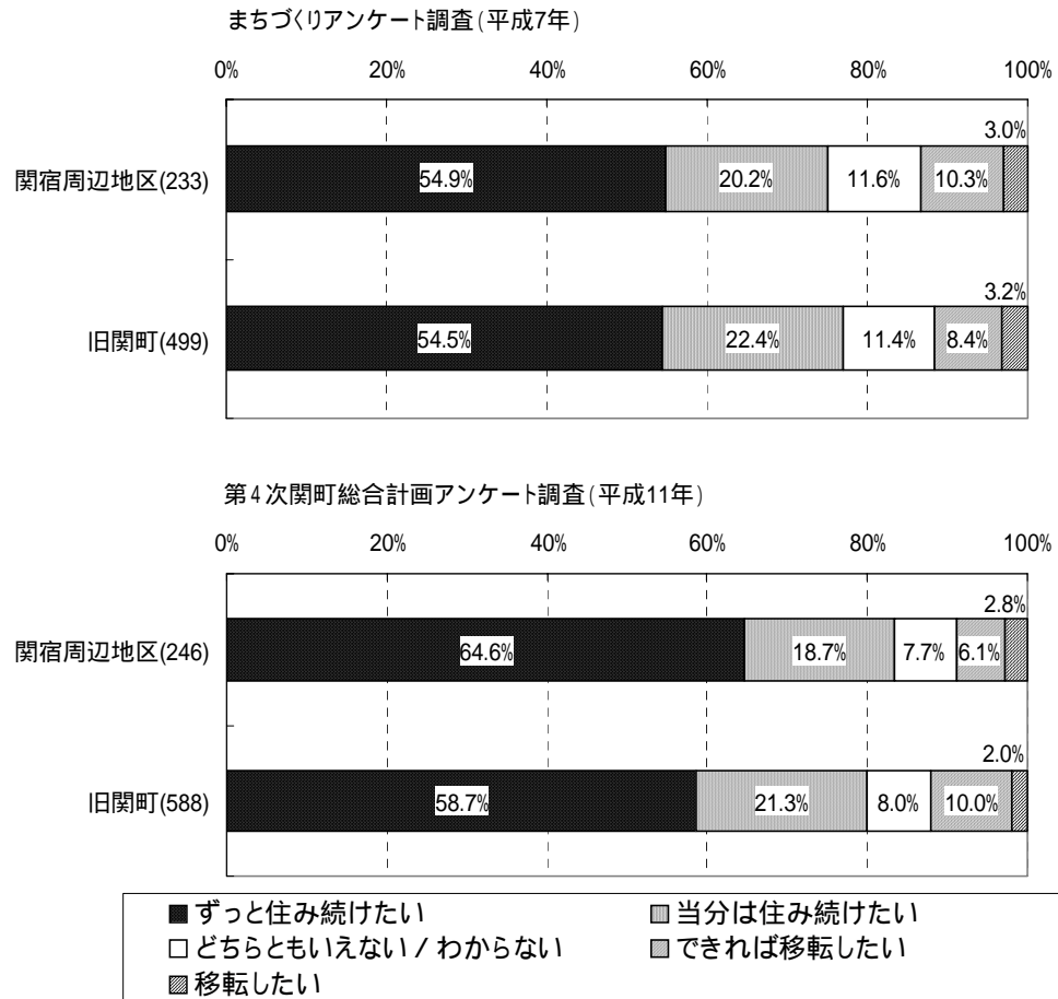
図 2-8 定住意向
