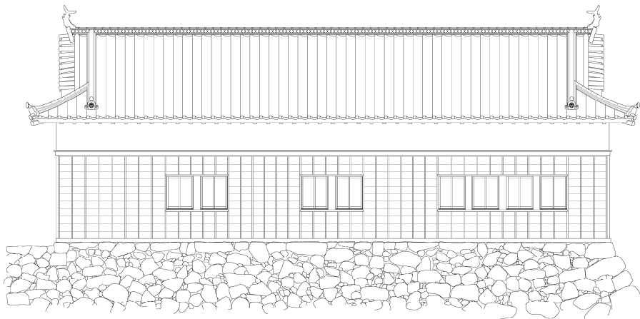
现状南立面图
