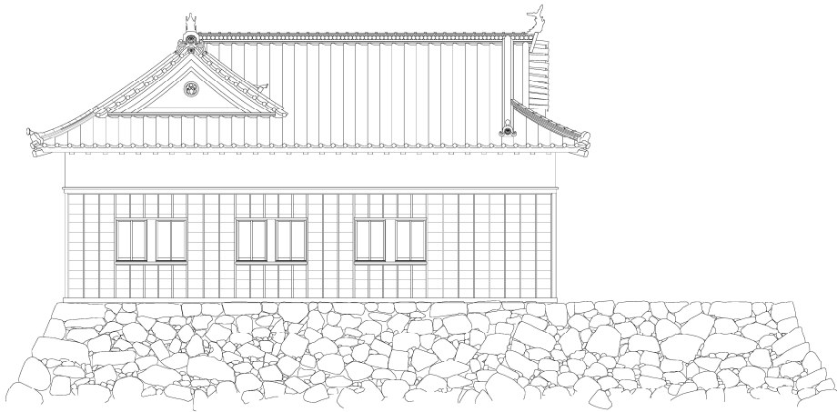
现状东立面图
