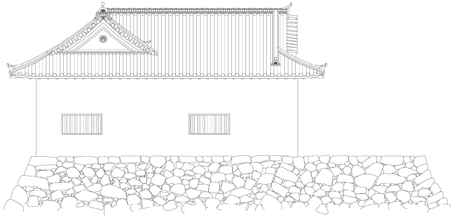
計画東立面図
