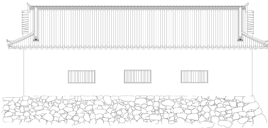
現状南立面図
