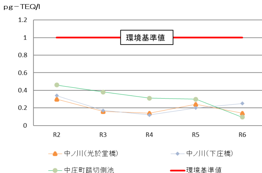
図6-2 水質②のダイオキシン類測定結果
