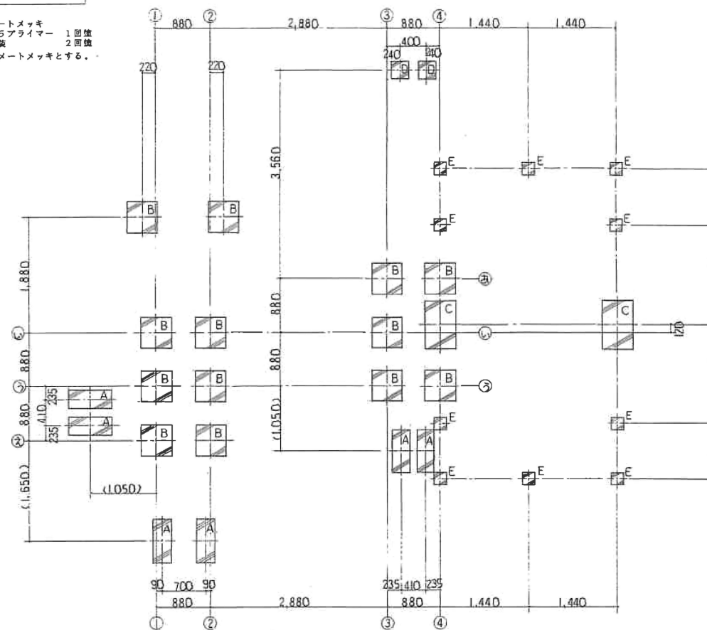
PG-540308 木製コンビネーション S=1:40
