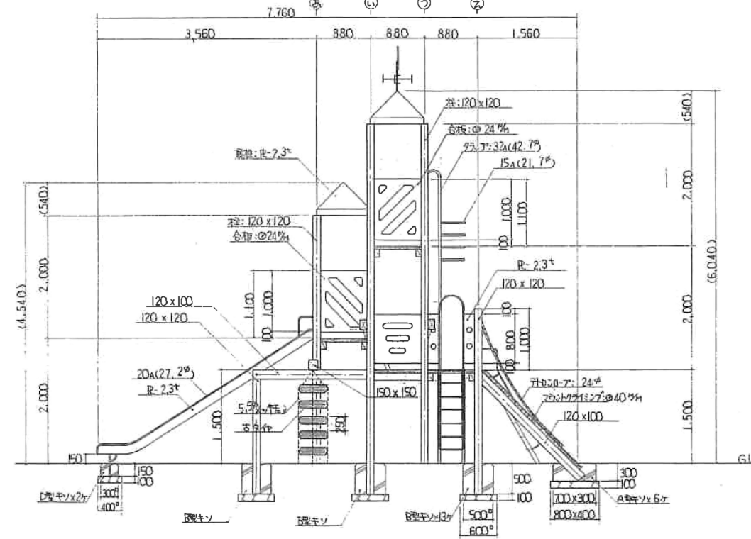
A方向矢視 S=1:40
