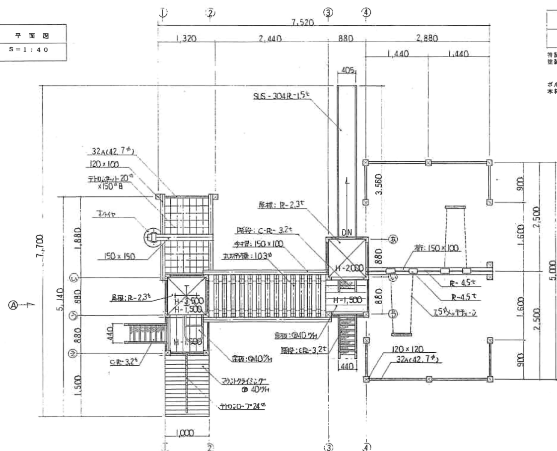
PG-540308 木製コンビネーション S=1:40
