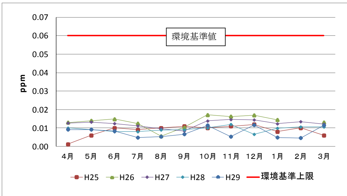
図 2-1-4 二酸化窒素の経月変化（神辺小学校）
