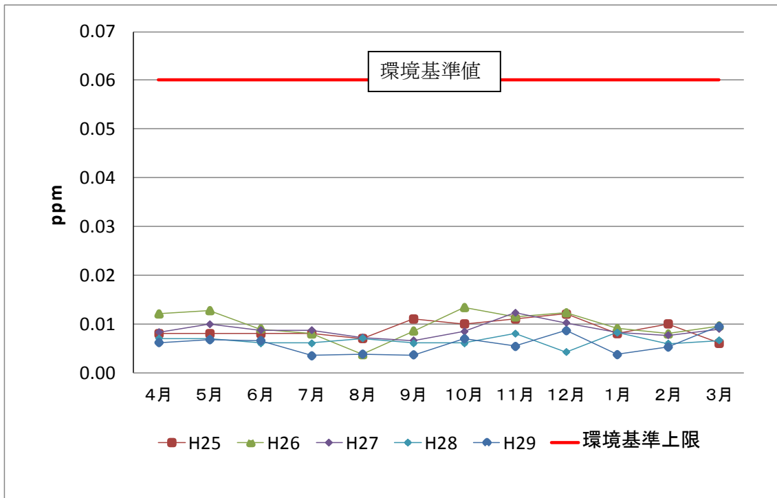
図 2-1-5 二酸化窒素の経月変化（昼生小学校）
