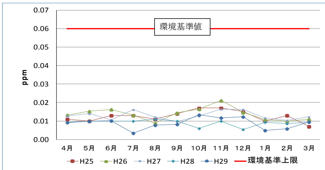
図2-1-1 二酸化窒素の経月変化（亀山市役所）
