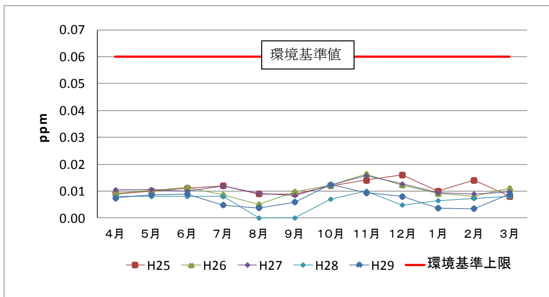
図2-1-2 二酸化窒素の経月変化（川崎小学校）
