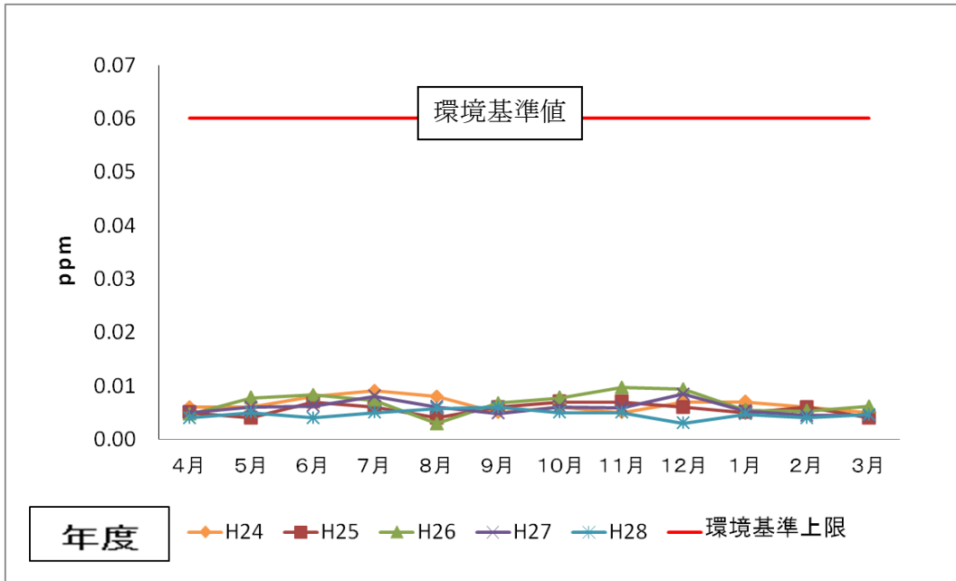
図 2-1-3 二酸化窒素の経月変化（白川小学校）
