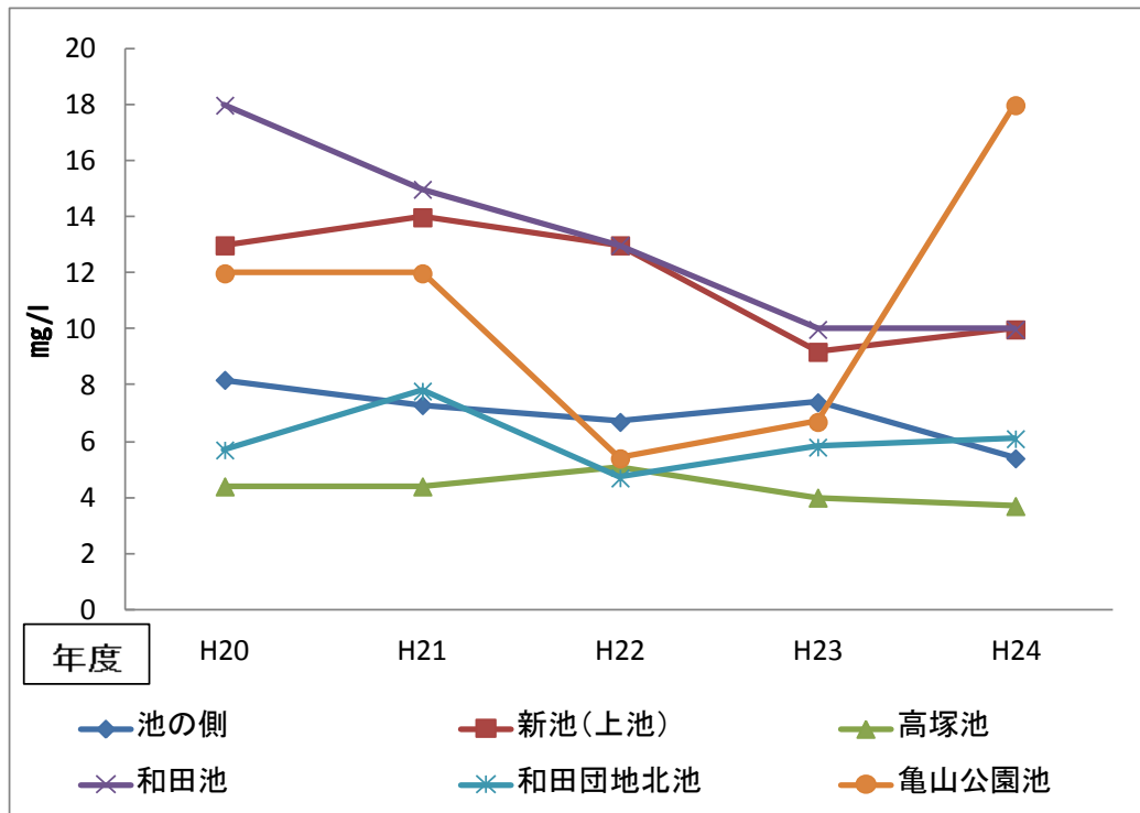
図 3－2 ため池のCOD 75%水質値の経年変化
