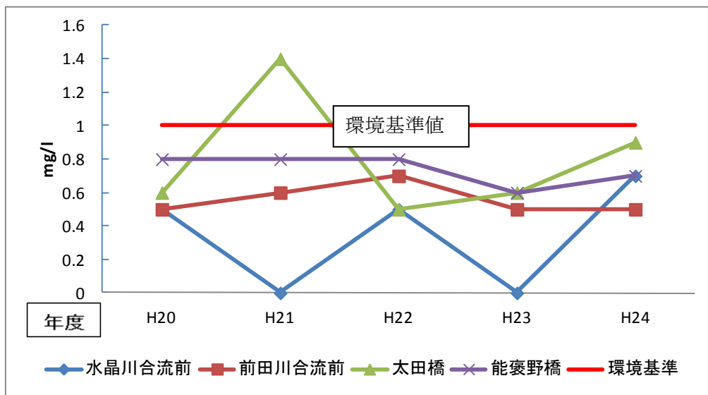
図 3-1-1 安楽川のBOD 75%水質値の経年変化
