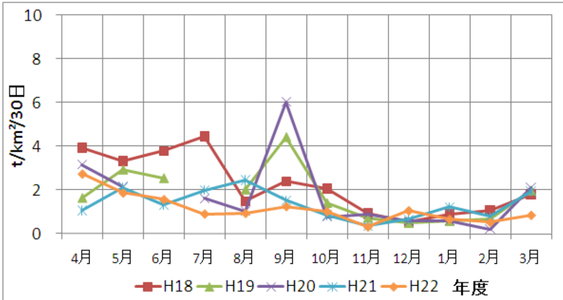
図 2-2-3 降下ばいじん総量の経月変化（昼生小学校）
