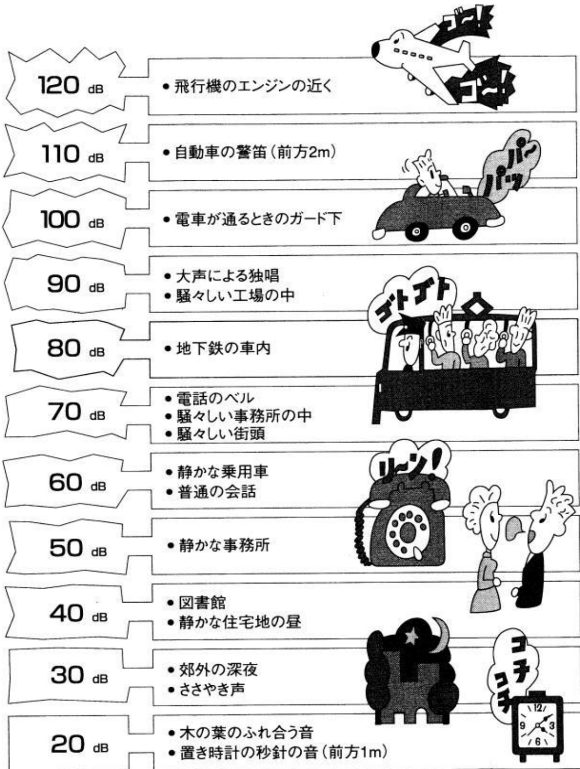
図4-2 騒音の大きさの例
