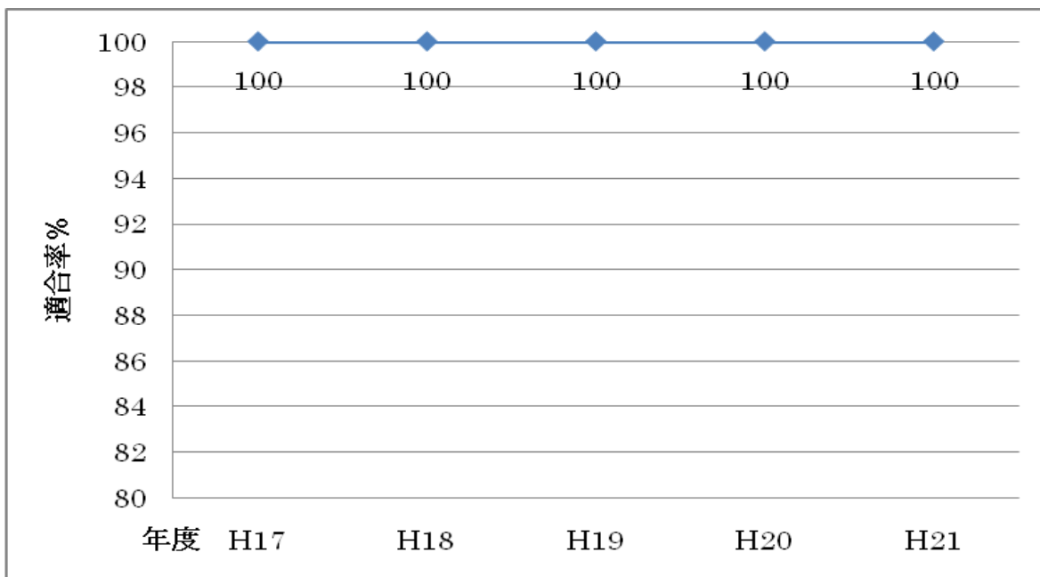
図4-3 道路交通環境基準適合状況
