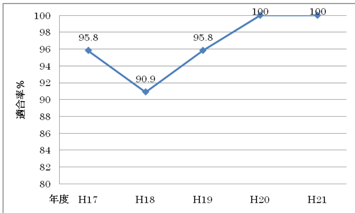
図4-1 環境騒音基準適合状況
