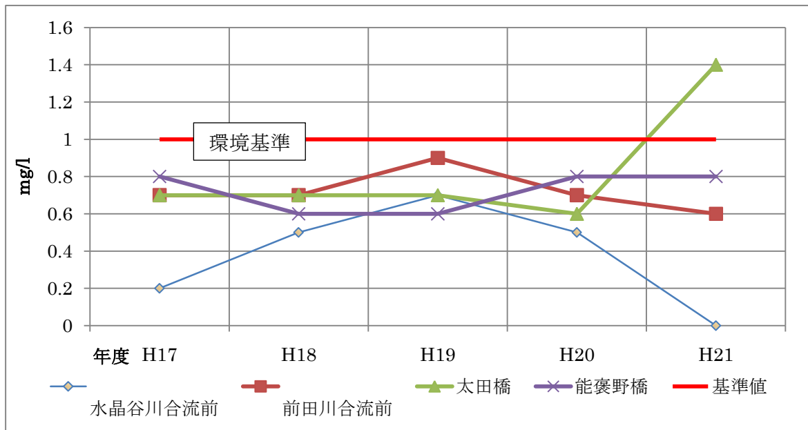
図3-1-1 一般河川のBOD75%水質値の経年変化（安楽川）
