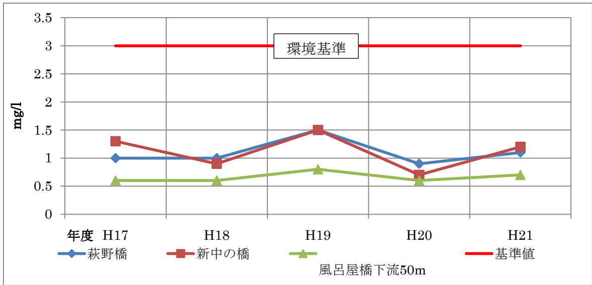
図3-1-3 一般河川のBOD75%水質値の経年変化(中ノ川)
