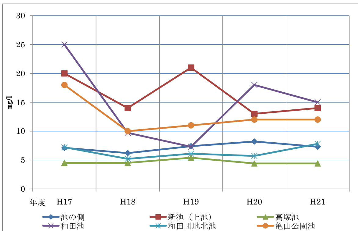
図3-2 ため池のCOD75%水質値の経年変化
