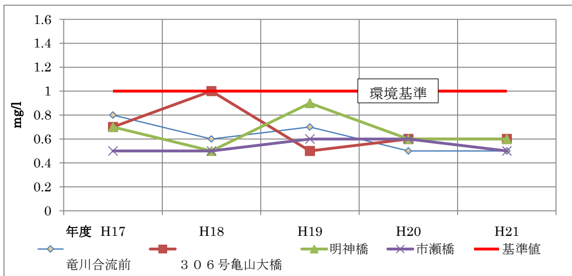
図3-1-2 一般河川のBOD75%水質値の経年変化（鈴鹿川）
