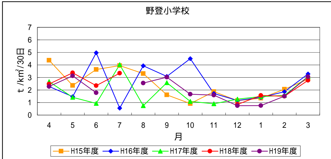
図2 - 2(2) 降下ばいじん総量の経月変化
