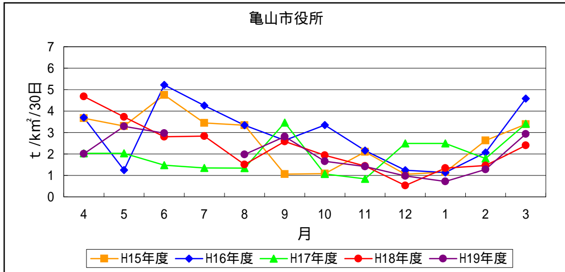
図2 - 2(1) 降下ばいじん総量の経月変化
