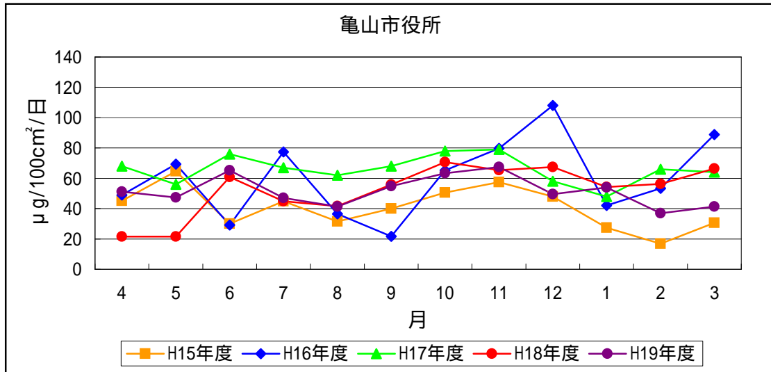
図2 - 1(1) 二酸化窒素の経月変化
