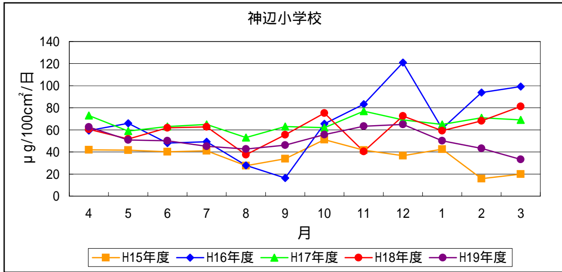
図2 - 1(2) 二酸化窒素の経月変化
