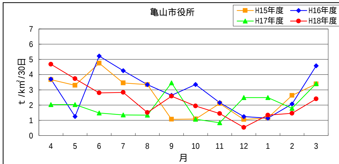
図3 - 2(1) 降下ばいじん総量の経月変化
