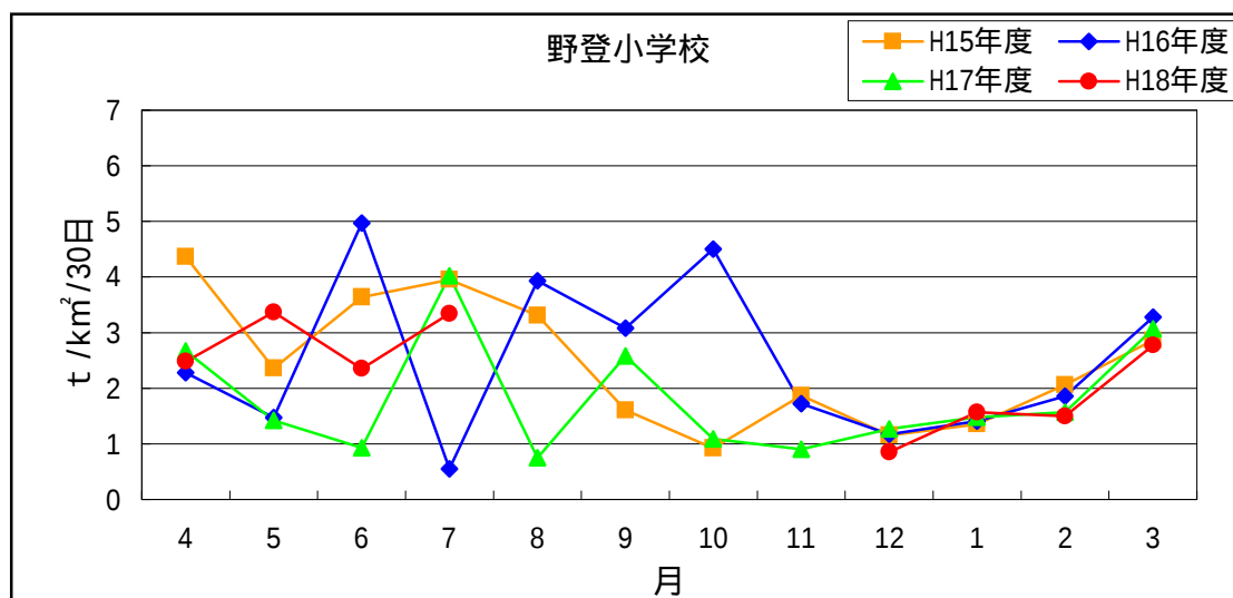
図3 - 2(2) 降下ばいじん総量の経月変化
