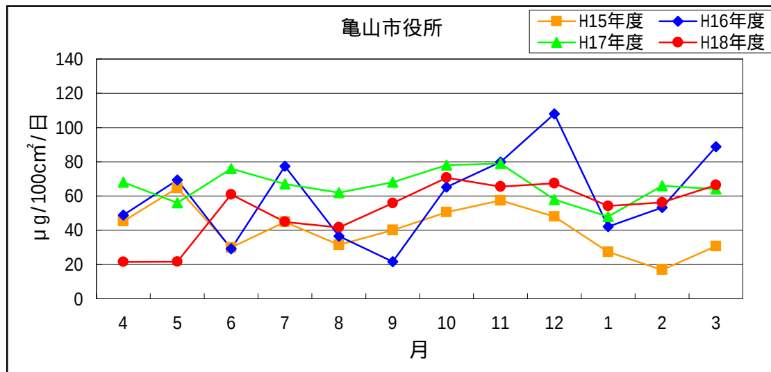
図3 - 1(1) 二酸化窒素の経月変化
