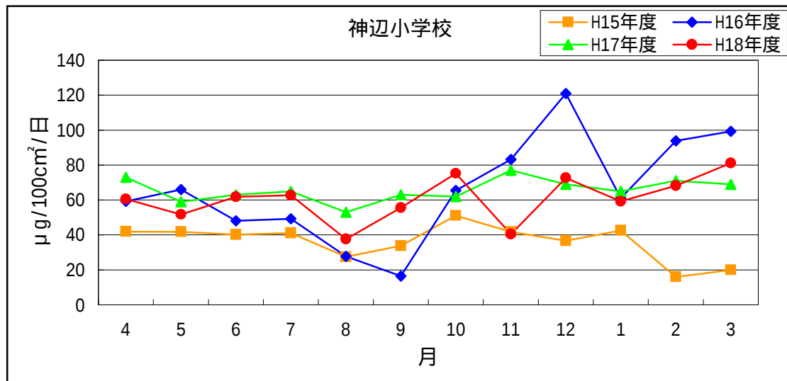
図3 - 1(2) 二酸化窒素の経月変化
