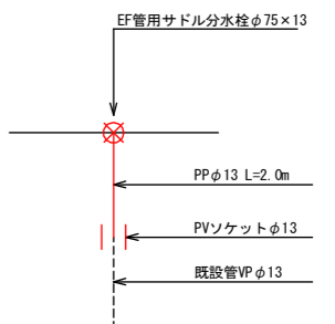
※S6 詳細図 N=2 L=2.0m×2=4.0m
