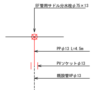
※S5 詳細図 N=1 L=4.5m×1=4.5m
