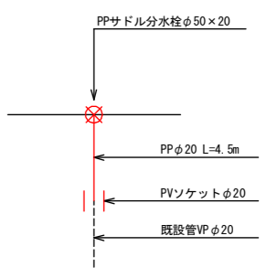
※S9 詳細図 N=1 L=4.5m×1=4.5m
