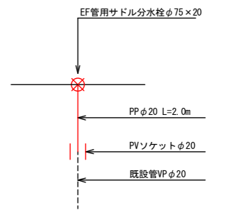
※S10 詳細図 N=1 L=2.0m×1=2.0m
