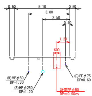
G-G'
