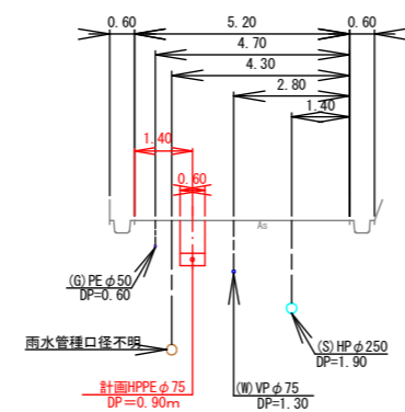
F-F'
