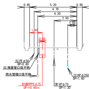
D-D'
