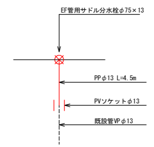
※S5 詳細図 N=7 L=4.5m×7=31.5m
