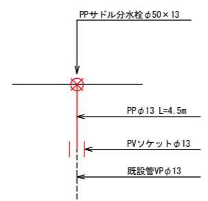
※S7 詳細図 N=4+6=10 L=4.5m×10=45.0m
