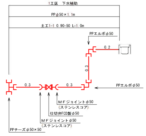
※排泥管 詳細図
