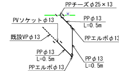
※8 仮設給水工詳細図 N=1
