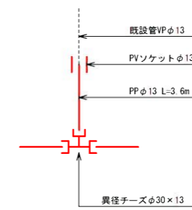
※1 詳細図
