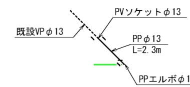
※11 仮設給水工詳細図 N=1
