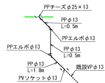
※9 仮設給水工詳細図 N=1
