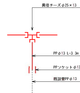
※1 詳細図
