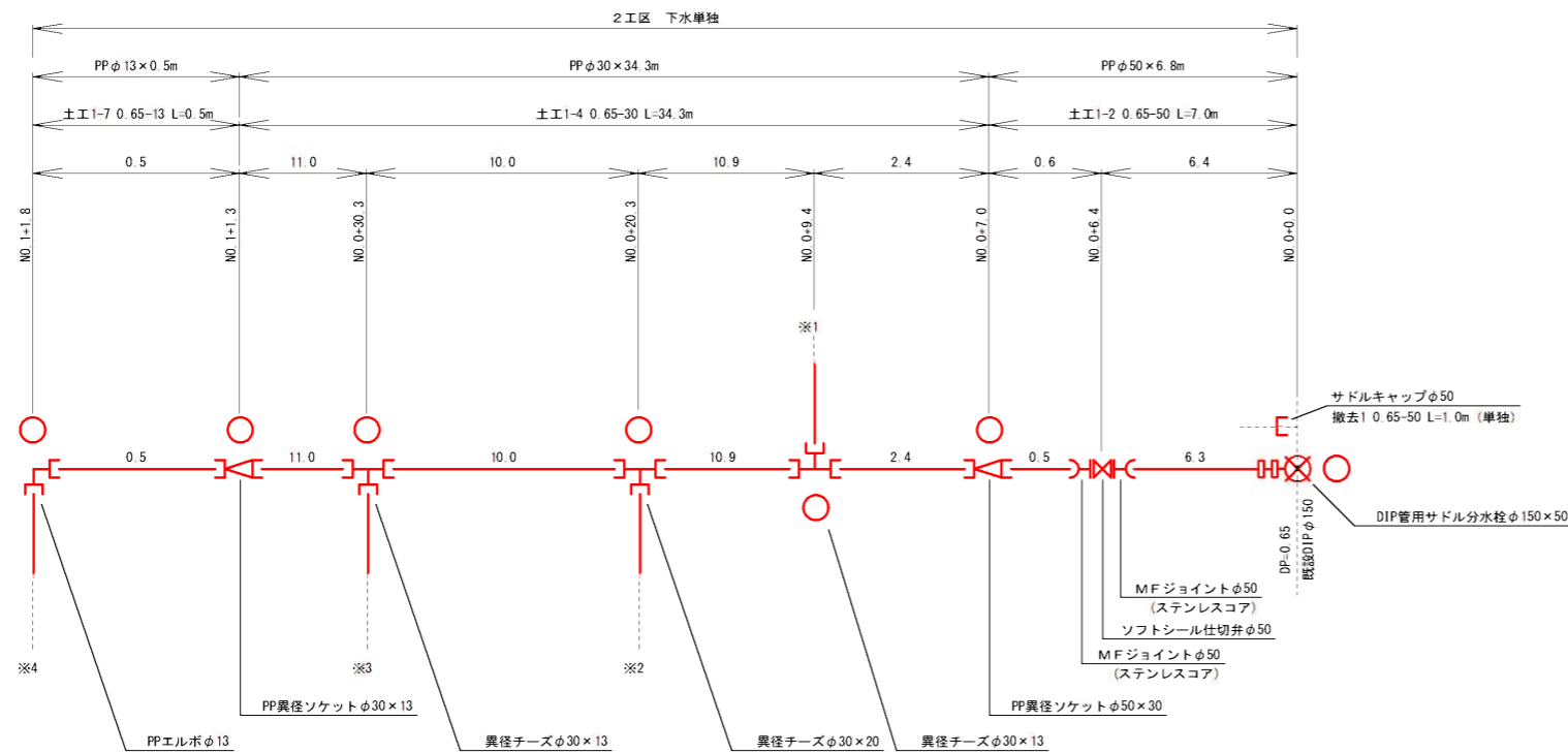
※3 詳細図
