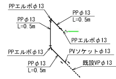
※4 仮設給水工詳細図 N=1
