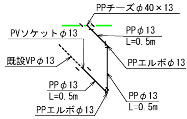
※1 仮設給水工詳細図 N=2
