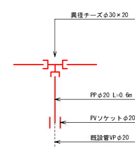
※2 詳細図
