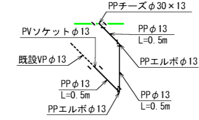
※7 仮設給水工詳細図 N=1
