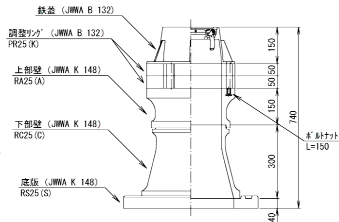
円形 1号 (H=900)
