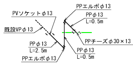
※3 仮設給水工詳細図 N=1
