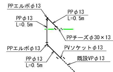
※2 仮設給水工詳細図 N=2
