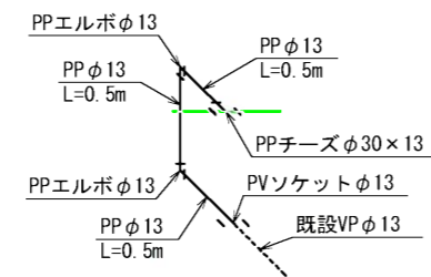
※6 仮設給水工詳細図 N=1
