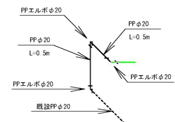
※2 仮設給水工詳細図
