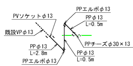
※5 仮設給水工詳細図 N=2
