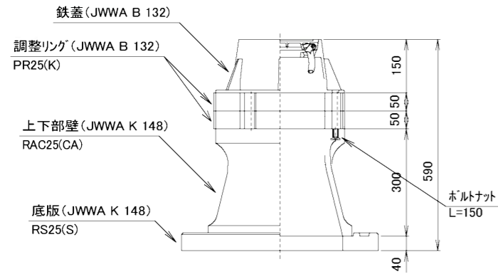
円形 1号 (H=600)
