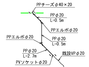
※12 仮設給水工詳細図 N=1
