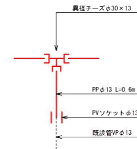
※3 詳細図
