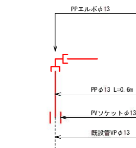
※4 詳細図
