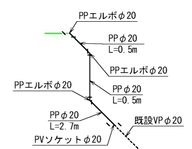
※13 仮設給水工詳細図 N=1
