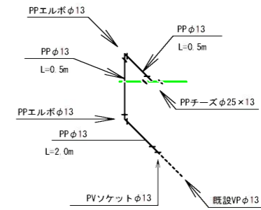
※1 仮設給水工詳細図 土工1-2 0.3-13 L=0.5m
