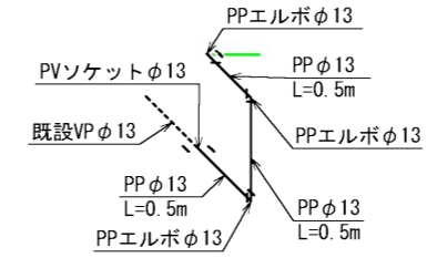
※10 仮設給水工詳細図 N=1
