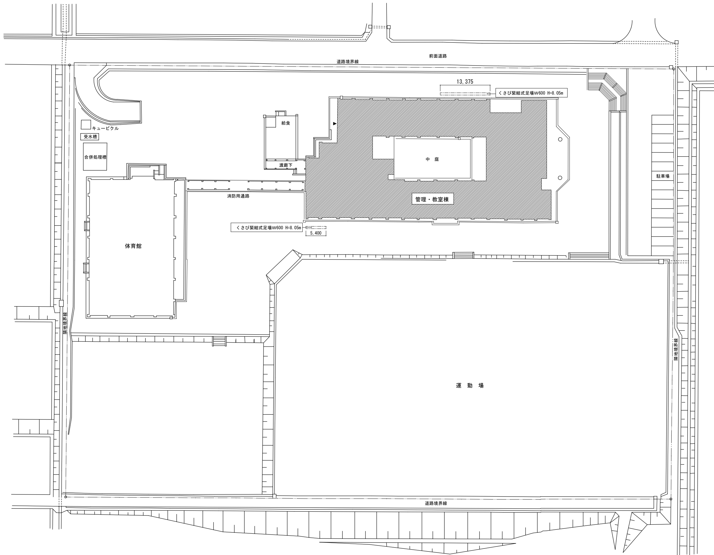
配置図 1/600
