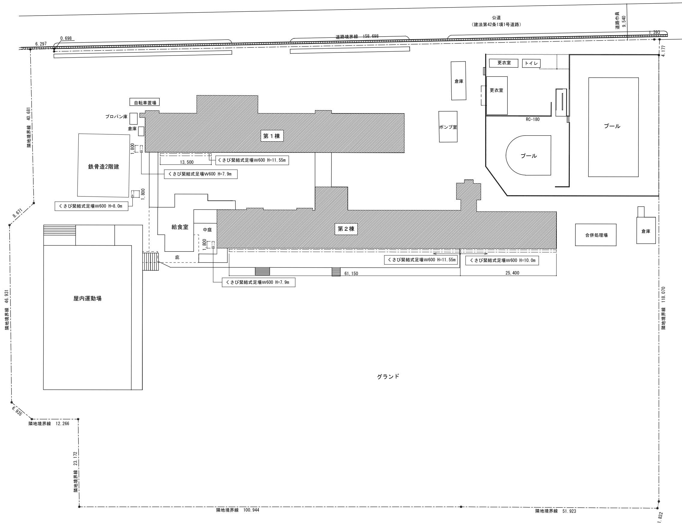
配置図 1/600
