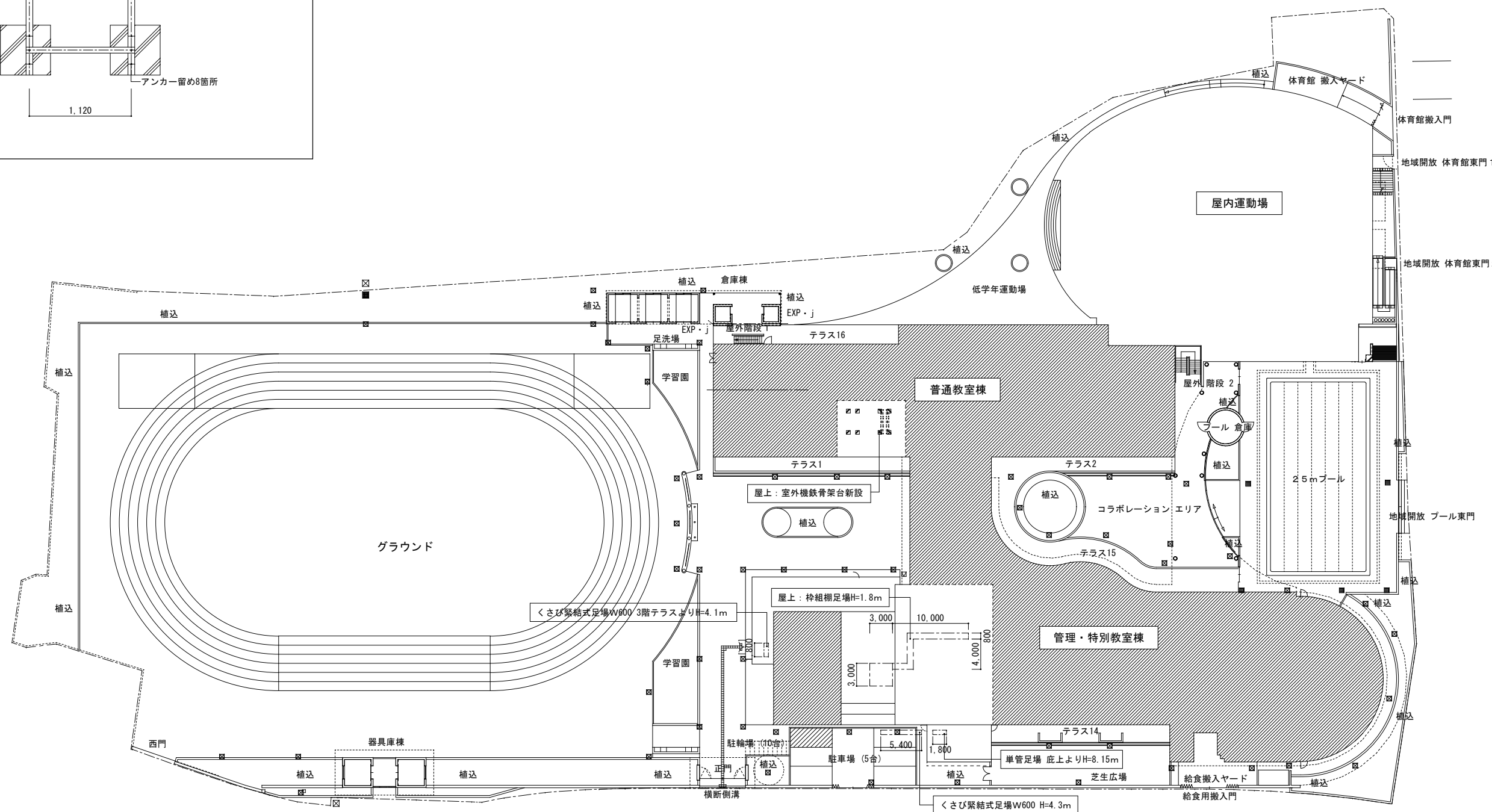
配置図 1/600
