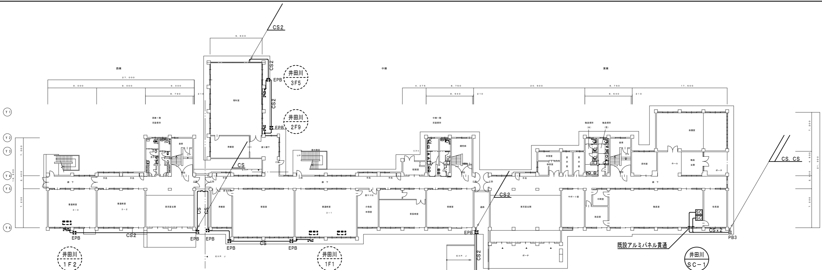
1階平面図
